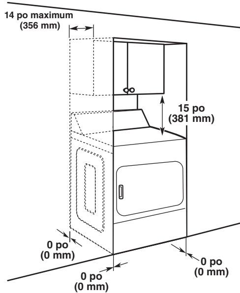
Vue d'avant, encastrement
