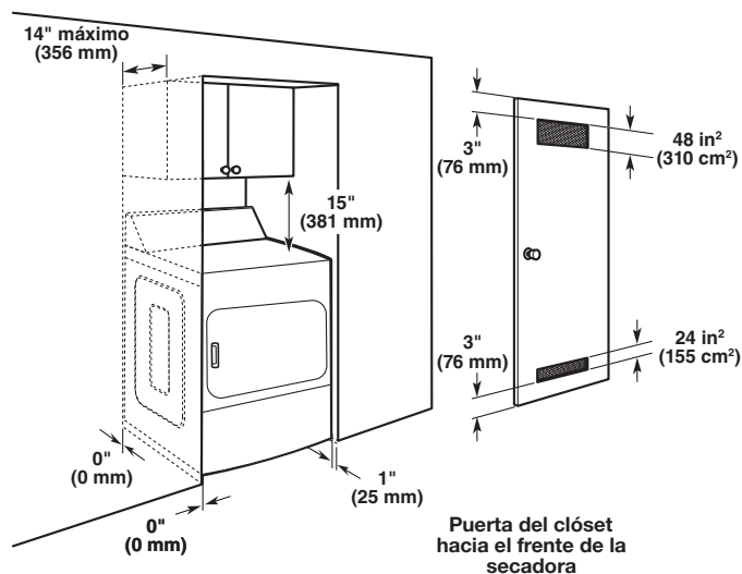
Vista lateral, Empotrada en clóset
