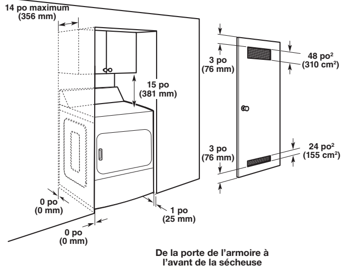
Vue latérale, encastrement dans une armoire
