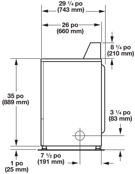
Vue latérale
