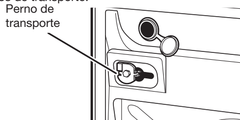
Perno de transporte con espaciador de plástico
