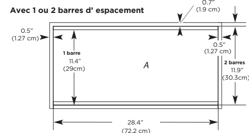
A. Ouverture dans le fond du placard
