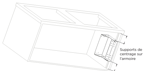
Position du support sans entretoises
