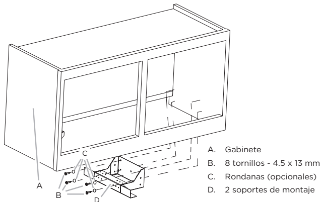
Orientación del soporte al gabinete de 36.7" (93.3cm)
