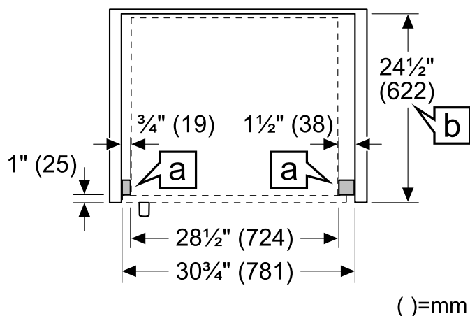
Vue de dessus porte battante droite
