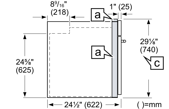
Vue latérale
