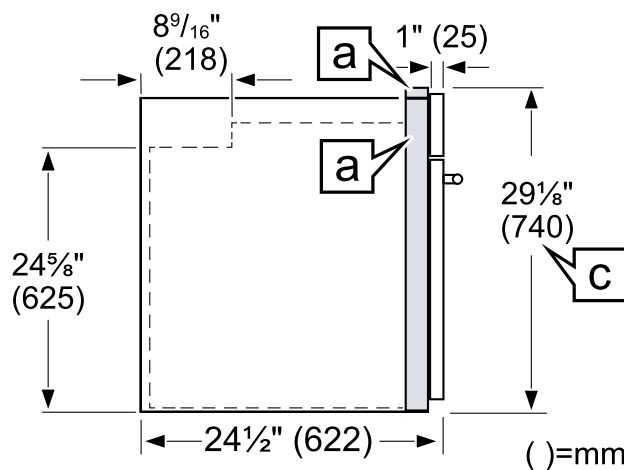
Vue latérale (représentative)
