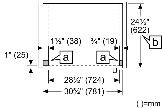
Top view left swing door
