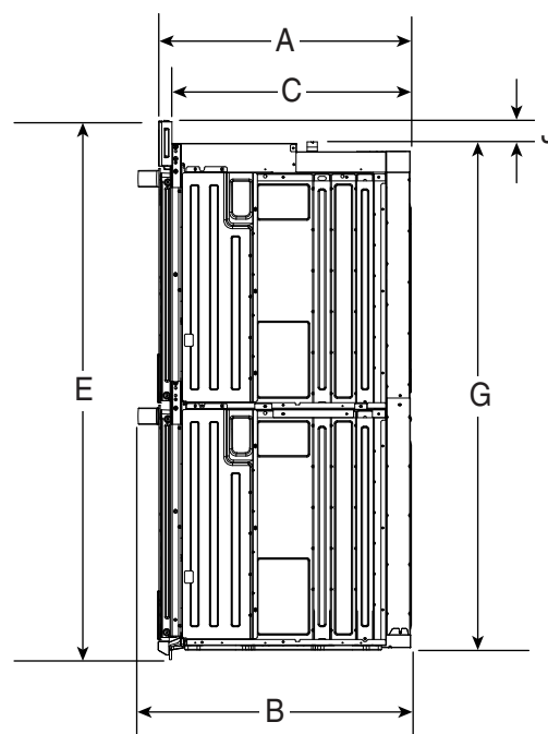
VUE LATÉRALE
