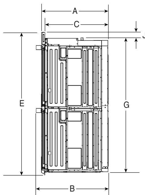
VISTA LATERAL
