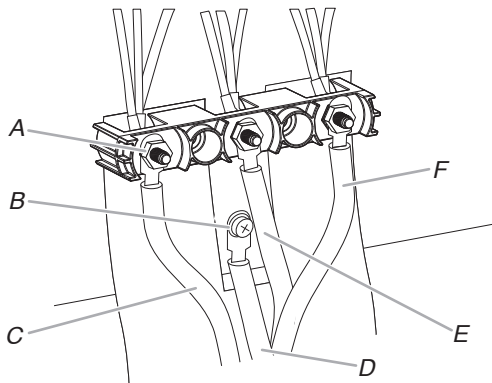
A. Écrou 10-32 à tête hexagonale B. Vis du fil de liaison à la terre C. Ligne 2 (rouge) D. Conducteur vert (liaison à la terre) E. Conducteur neutre (centre) F. Ligne 1 (noir)
