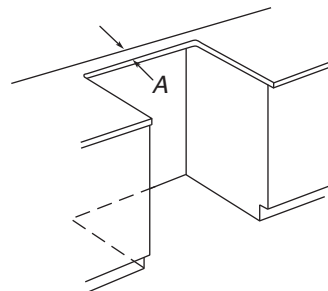
A. Épaisseur du mortier pour comptoir
