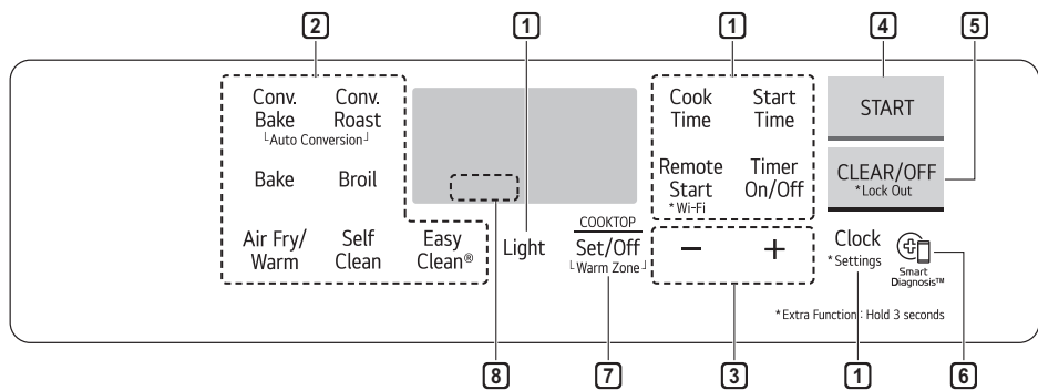
Modelo LREL6323*
