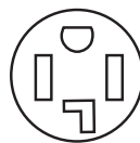
Tomacorriente de 4 hilos (14R-30R)
