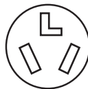
Prise murale à 3 conducteurs (10R-30R)
