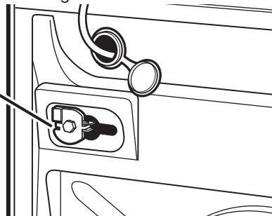
Boulon d'expédition
