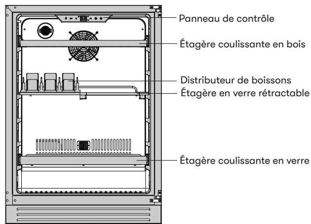
PRPB24C01CG sans porte et avec distributeur de boissons et étagère en verre rétractable
