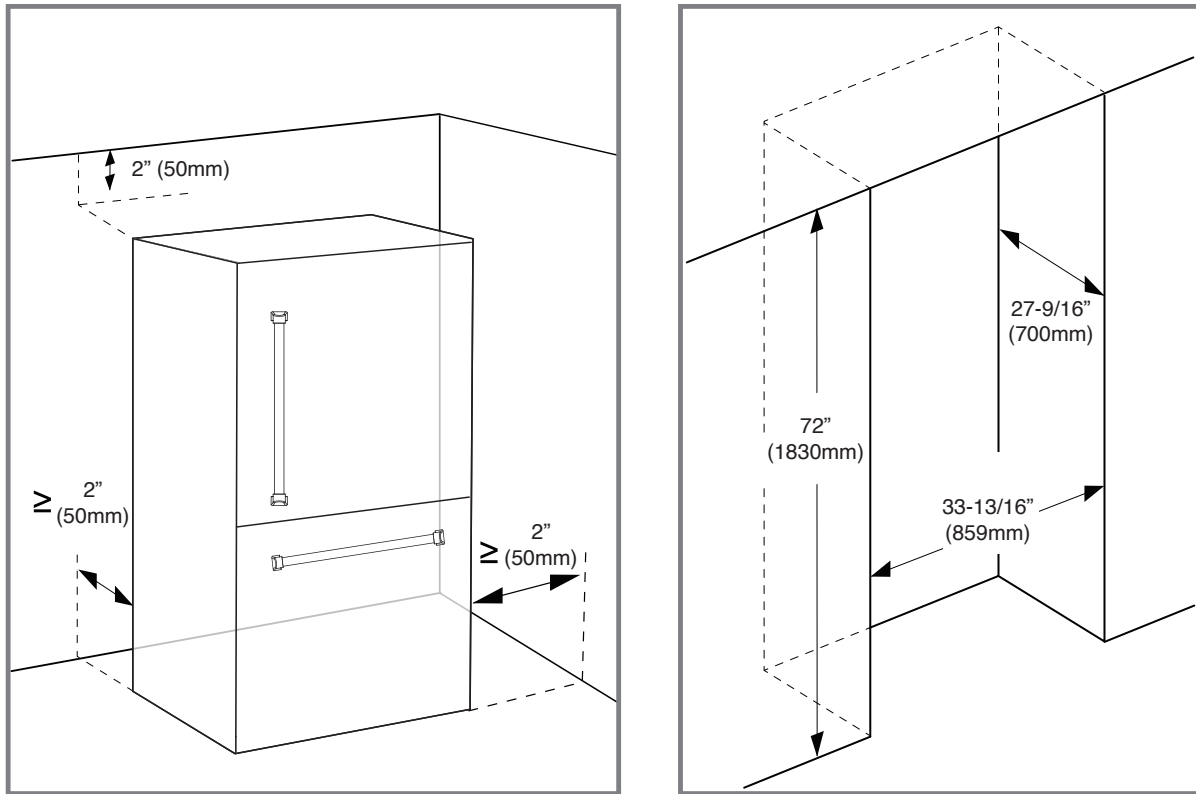
Cutout Dimensions
