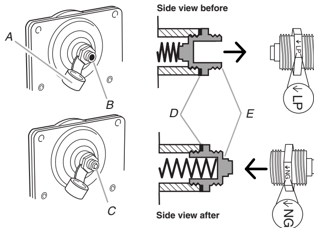
A. Capuchon en plastique B. Capuchon du détenteur; extrémité creuse ouverte vers l'extérieur C. Capuchon du détenteur; extrémité borgne vers l'extérieur D. Rondelle E. Capuchon du détenteur
