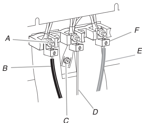
A. Écrou hexagonal 10-32 B. Ligne 2 (rouge) C. Vis de liaison à la terre D. Fil de mise à la terre nu (vert) E. Ligne 1 (noir) F. Cousse
