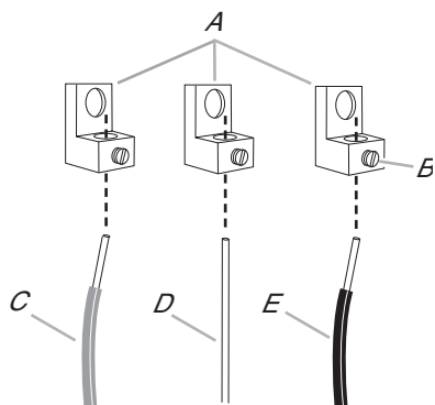
A. Cousse B. Vis de blocage C. Conducteur de ligne 2 (rouge) D. Fil de mise à la terre nu (vert) E. Conducteur de ligne 1 (noir)
