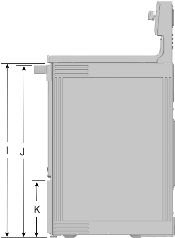
VISTA LATERAL
