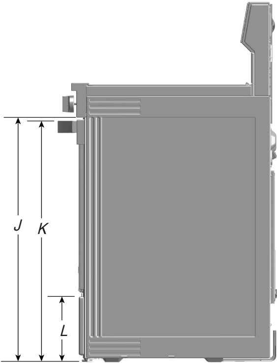
VUE LATÉRALE
