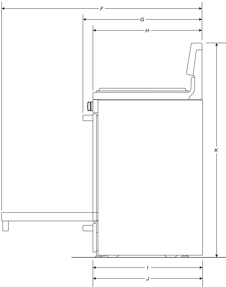
VUE LATÉRALE
