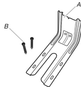
A. Bride antibascullement B. #12 x 1 5/8" (4,1 cm) Vis (2)
