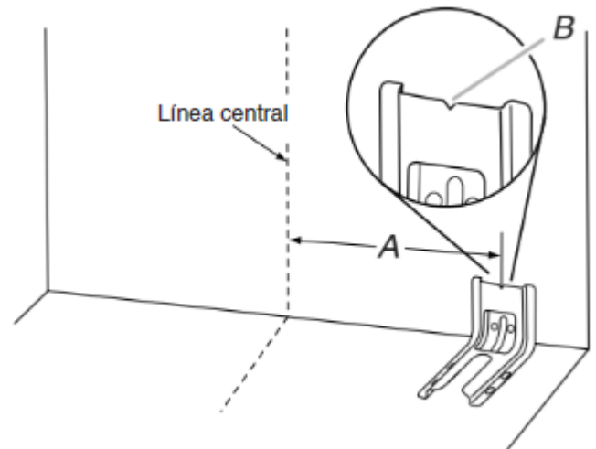
A. 12 \frac{9}{16} " (31,9 cm)
