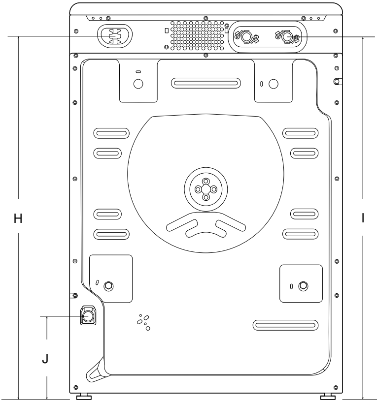
VUE ARRIÈRE
