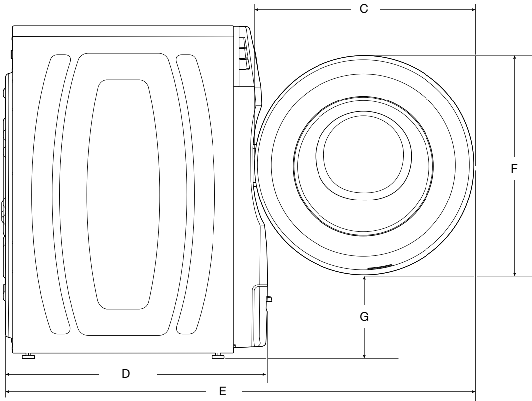
VUE LATÉRALE
