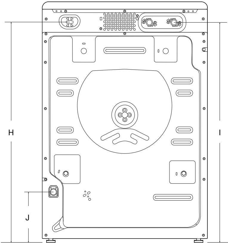
VISTA POSTERIOR
