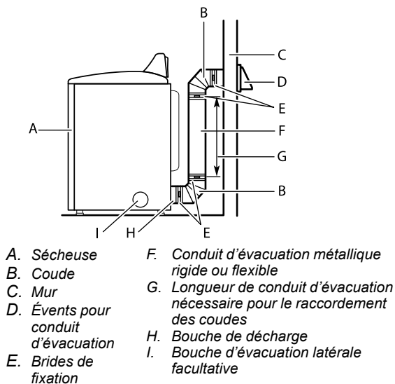
Installation au-dessus de la sècheuse Installation en périscope (également disponible avec un coude décalé)
