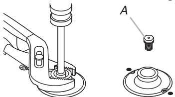
A. Tornillo de orificios de gas propano
