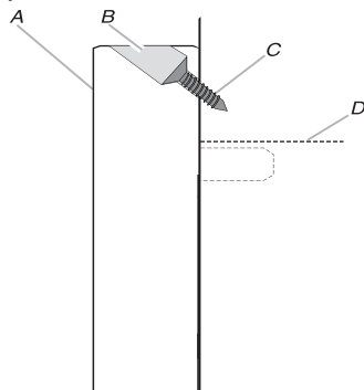
A. Marco del kit de molduras B. Guía del orificio de montaje C. Tornillo de cabeza plana para madera n.º 7-16 x 15/16" (4) D. Parte superior del recorte
