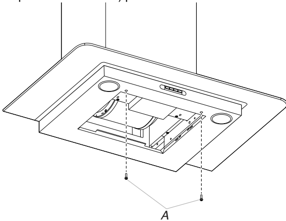
A. Vis T20® de 4,2 x 8 mm
