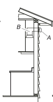
A. Bouche de décharge murale B. Conduit rond de 6 po (15,2 cm)
