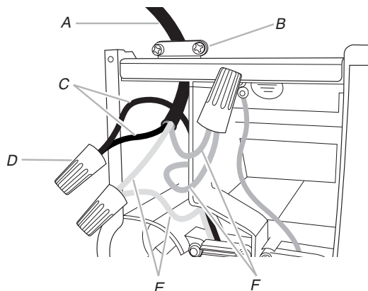
A. Câble d'alimentation électrique du domicile B. Serre-câbles (homologation UL ou CSA) C. Conducteurs noirs D. Connecteurs de fils (homologation UL) E. Conducteurs blancs F. Conducteurs verts (ou nus) et vert jaune de liaison à la terre
