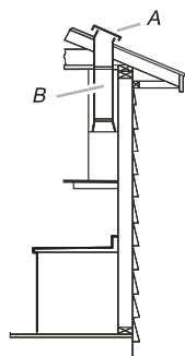
A. Bouche de décharge sur toit B. Conduit rond de 6 po (15,2 cm)
