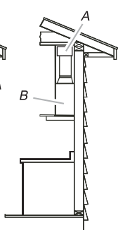
A. Déflecteur B. Conduit rond de 6 po (15,2 cm)
