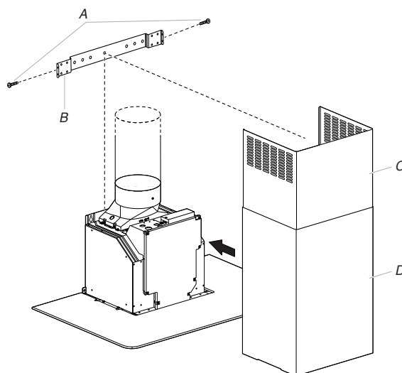
A. Vis de 4,2 x 8 mm B. Support
