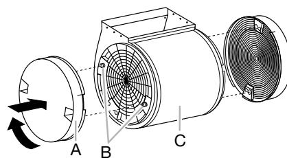
A. Filtres à charbon
